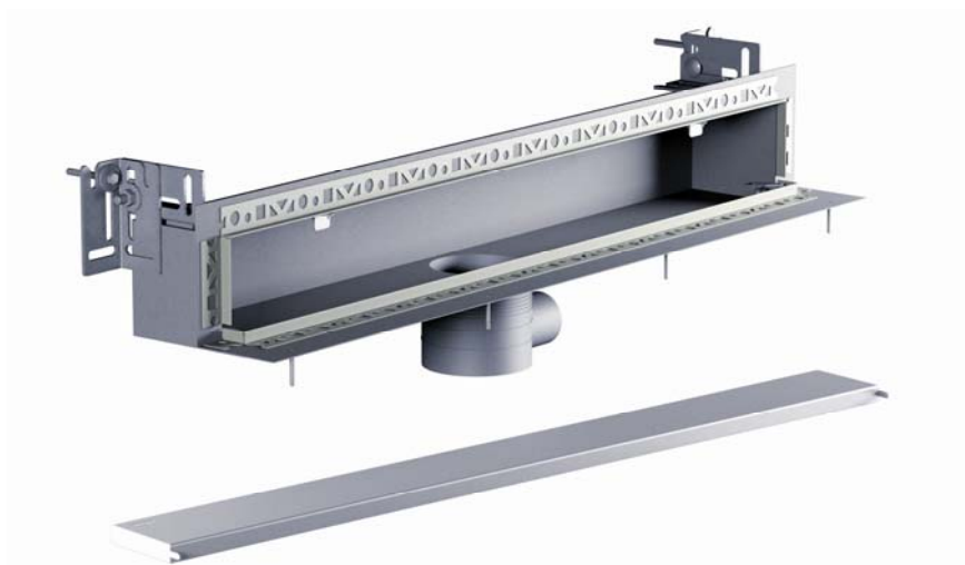
Die „TersoWALL“ Duschrinne zur Wandmontage
